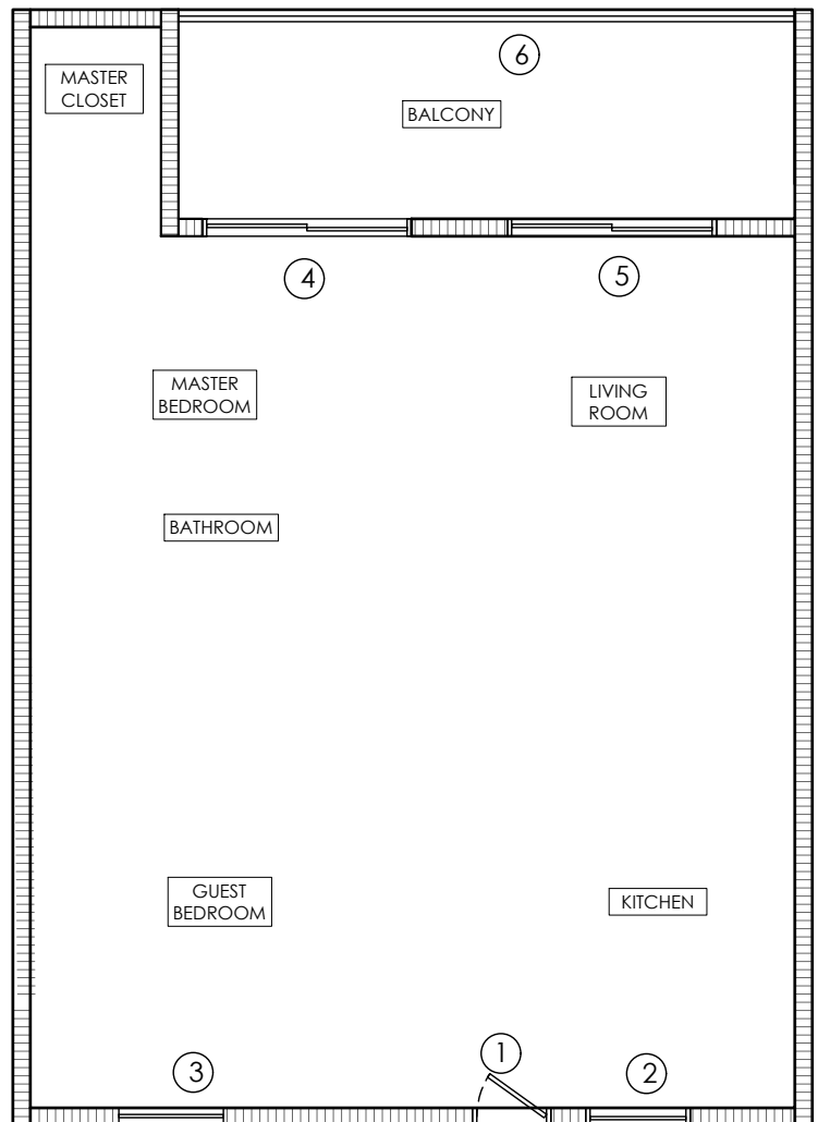
FLOOR PLAN SCALE: 1/8" = 1'-0"
